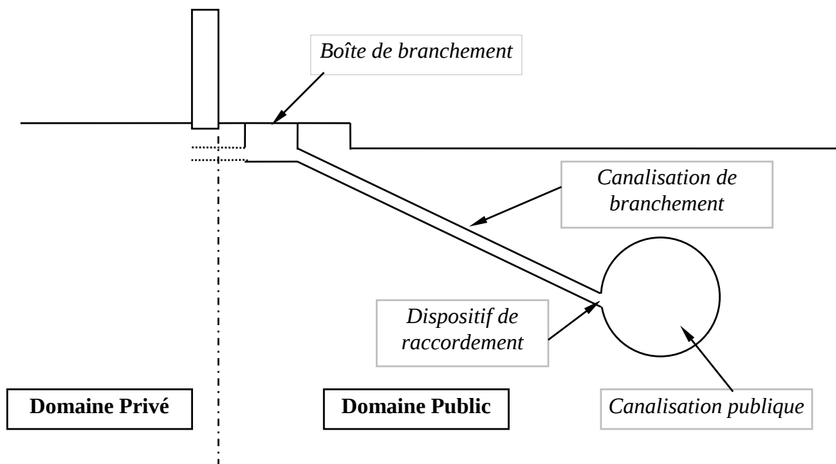
Figure 1. Description schématique d'un branchement
